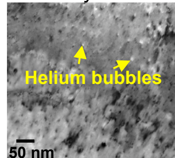
Pure Cu
